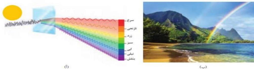
شکل ۱۴-ا) نور خورشید هنگام عبور از منشور تجزیه می شود. ب) رنگین کمان، گستره‌ای از رنگ‌های سرخ تا بنفش را در برمی گیرد.
